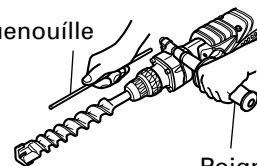
Poignée latérale
