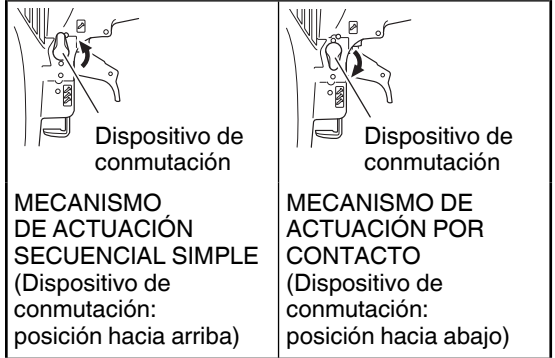
Dispositivo de conmutación para la operación de clavado
