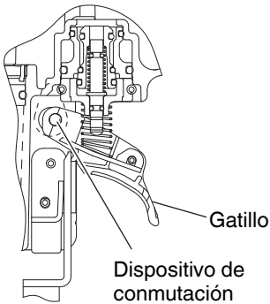
Vista ampliada de la parte de la válvula
